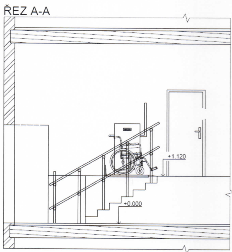
Obr. 1. Řez schodištěm s vyobrazením plošiny
